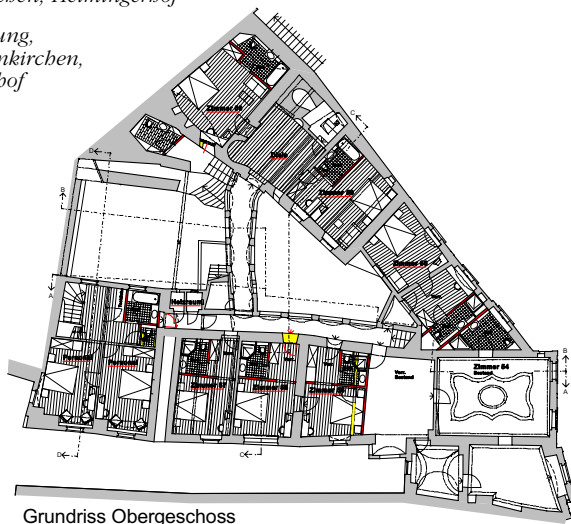
Grundriss Obergeschoss
