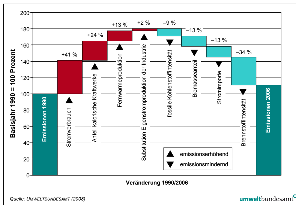
Abbildung 21: Komponentenzerlegung des Emissionstrends von Kohlendioxid aus dem Sektor Energieaufbringung.
