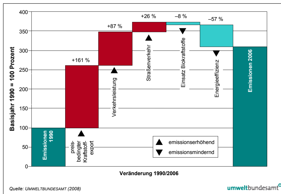
Abbildung 36: Komponentenzersetzung des Emissionstrends von Kohlendioxid im Bereich Güterverkehr.
