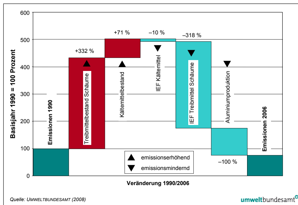
Abbildung 47: Komponentenzersetzung des Emissionstrends im Sektor F-Gase in Kohlendioxid-Äquivalenten.
