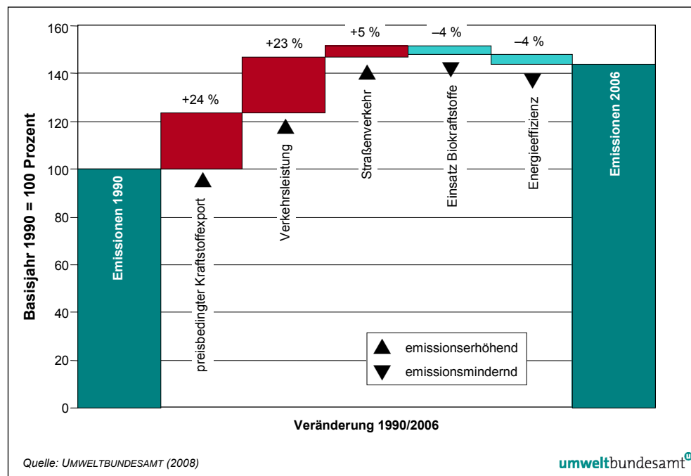
Abbildung 34 Komponentenzzerlegung des Emissionstrends von Kohlendioxid im Bereich Personenverkehr.
