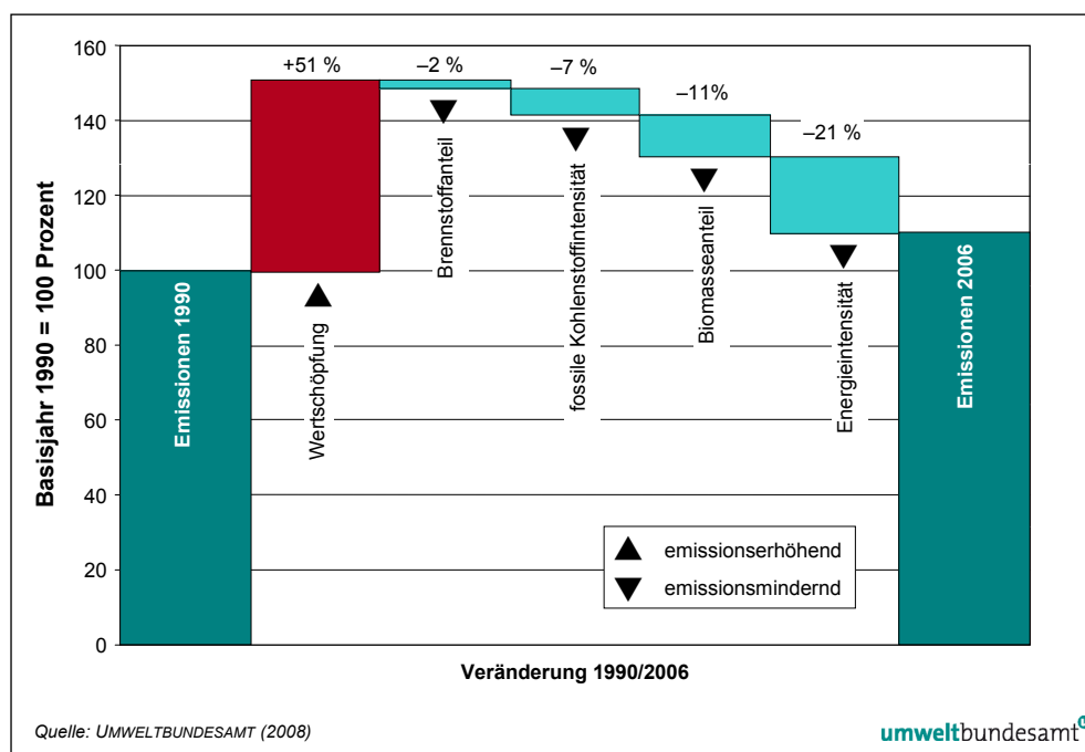
Abbildung 40: Komponentenerlegung des Emissionstrends von Kohlendioxid im Sektor Industrie und produzierendes Gewerbe (ohne Eisen- und Stahlerzeugung).
