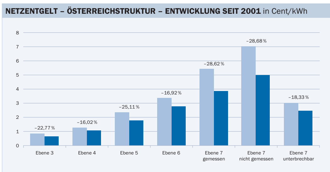
Abbildung 22 Entwicklung der Netzentgelte Strom seit 2001
