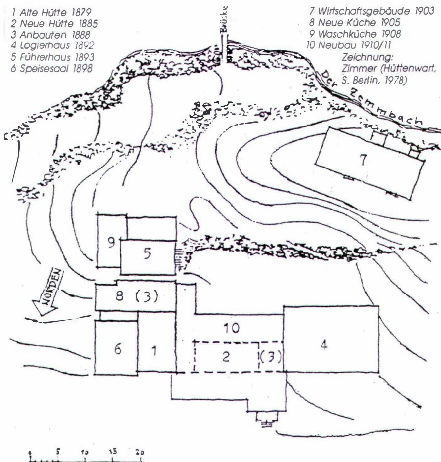
Abb. 2: Bauphasen Berlinerhütte
