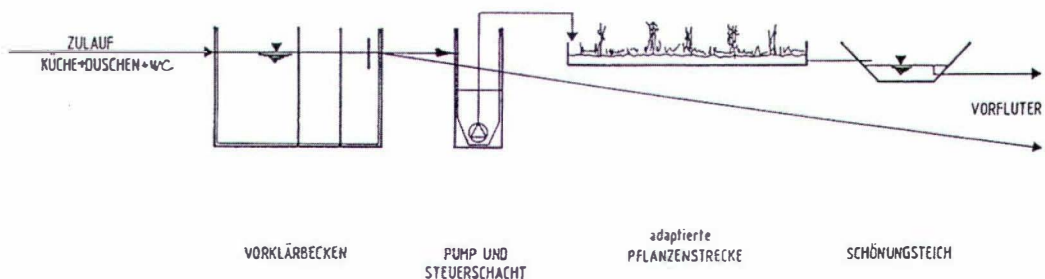
Abb. 41: Abwasserreinigungsanlage Dr.-Josef-Mehrl-Hütte
