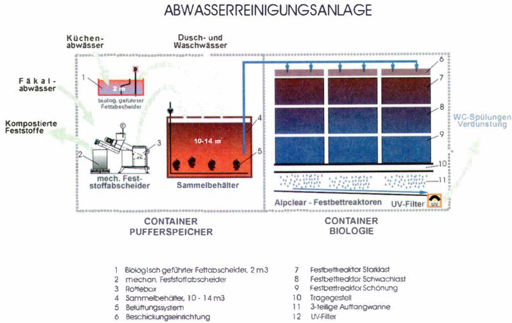
Abb. 58: Abwasserreinigungsanlage (Schema)
