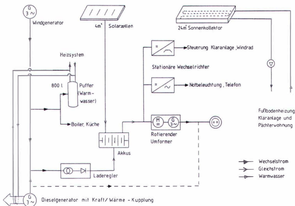
Abb. 70: Energieversorgung (Schema)
