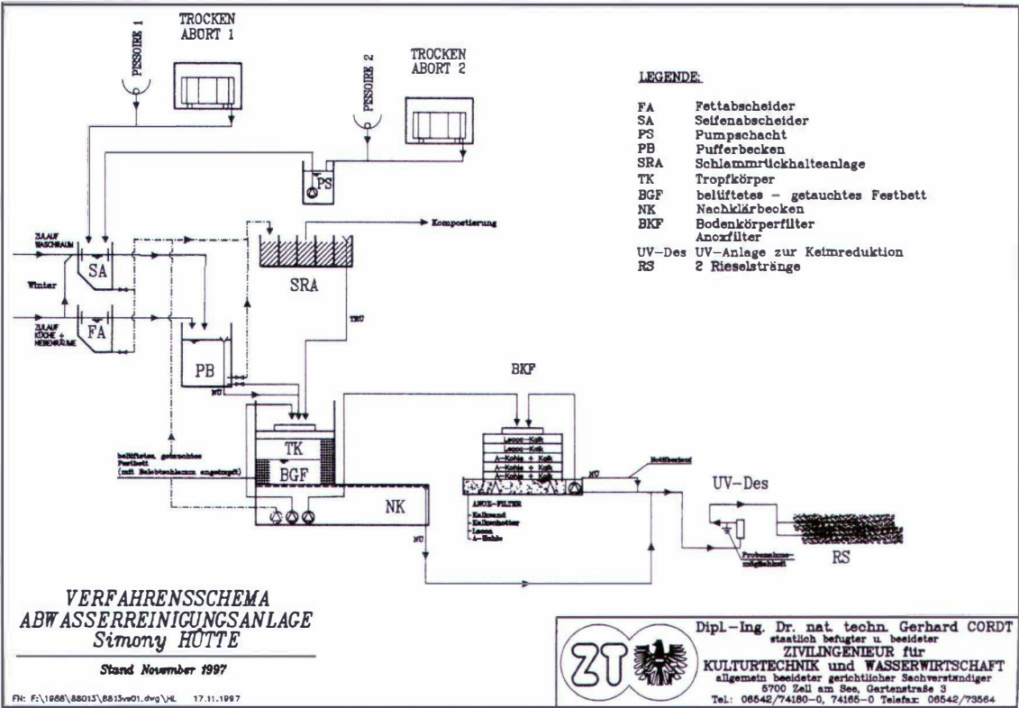
Abb. 72: Abwasserreinigungsanlage (Schema)
