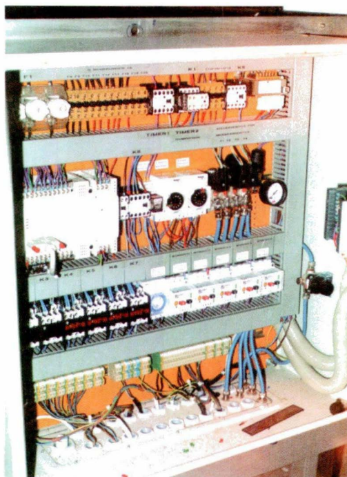
Abb. 7: Steuerung für Biologiestufe der Kläranlage (Wiesberghaus)
