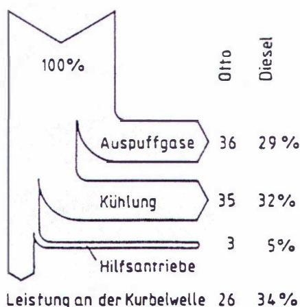
Abb. 14: Energieverteilung im Verbrennungsmotor
