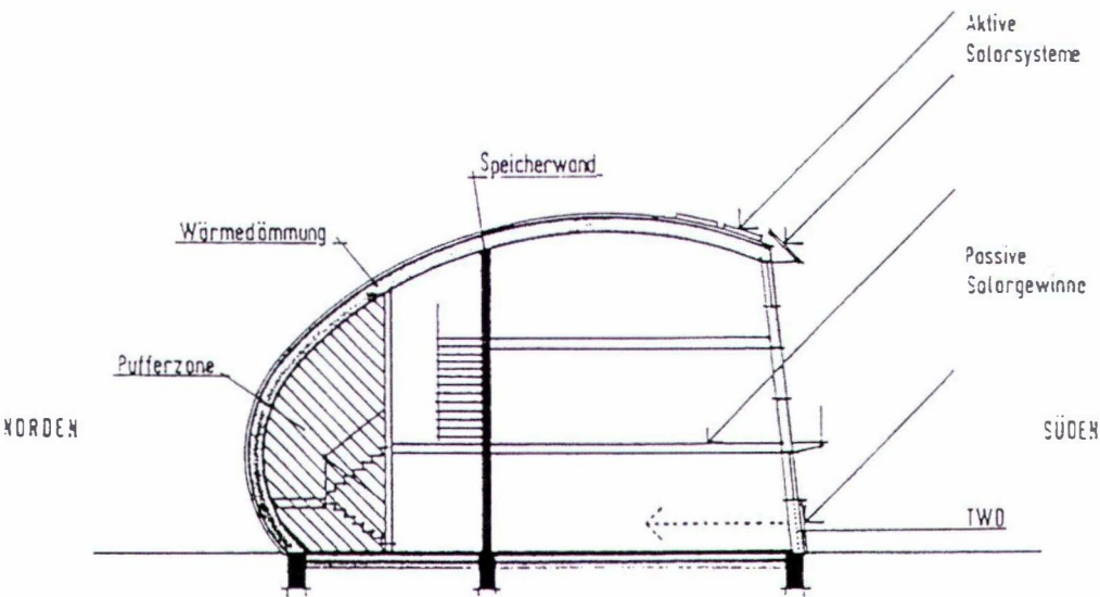
Abb. 23: Neue Stüdl Hütte (Schnitt)
