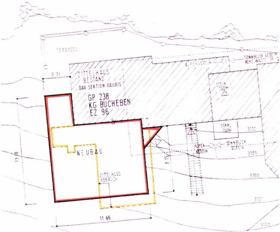
Abb. 77: Umbau: Grundriß
