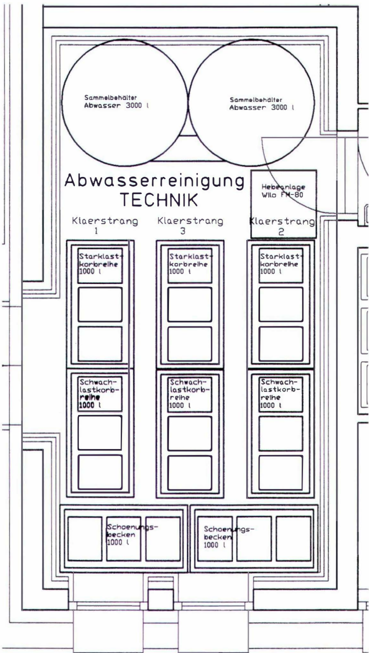
Abb. 79: Abwasserreinigungsanlage (Schema)
