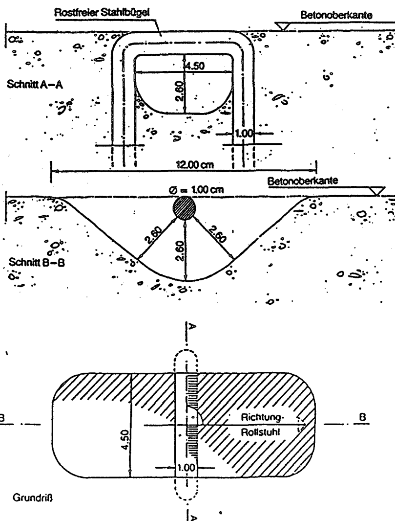
B: Befestigungsanker/Detail
