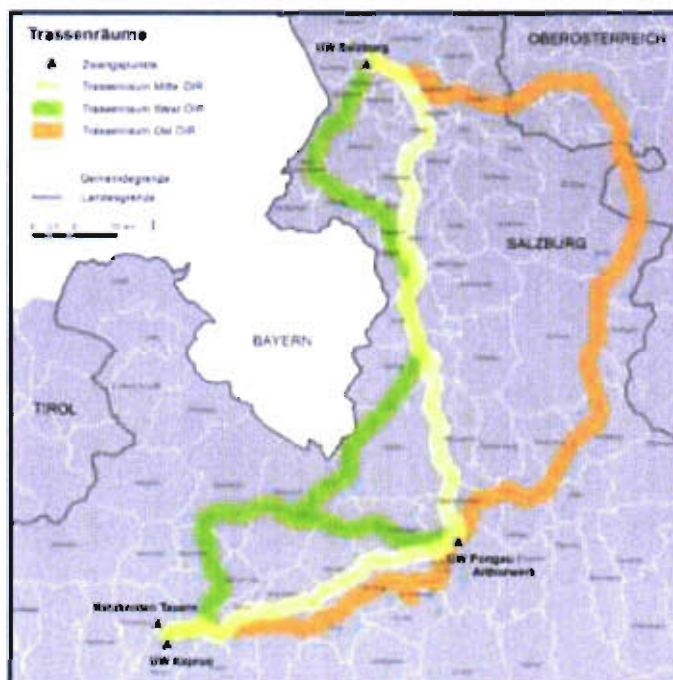
Abbildung 2-2: Auswahl alternativer Trassenräume, Quelle: OIR Studie 2006
