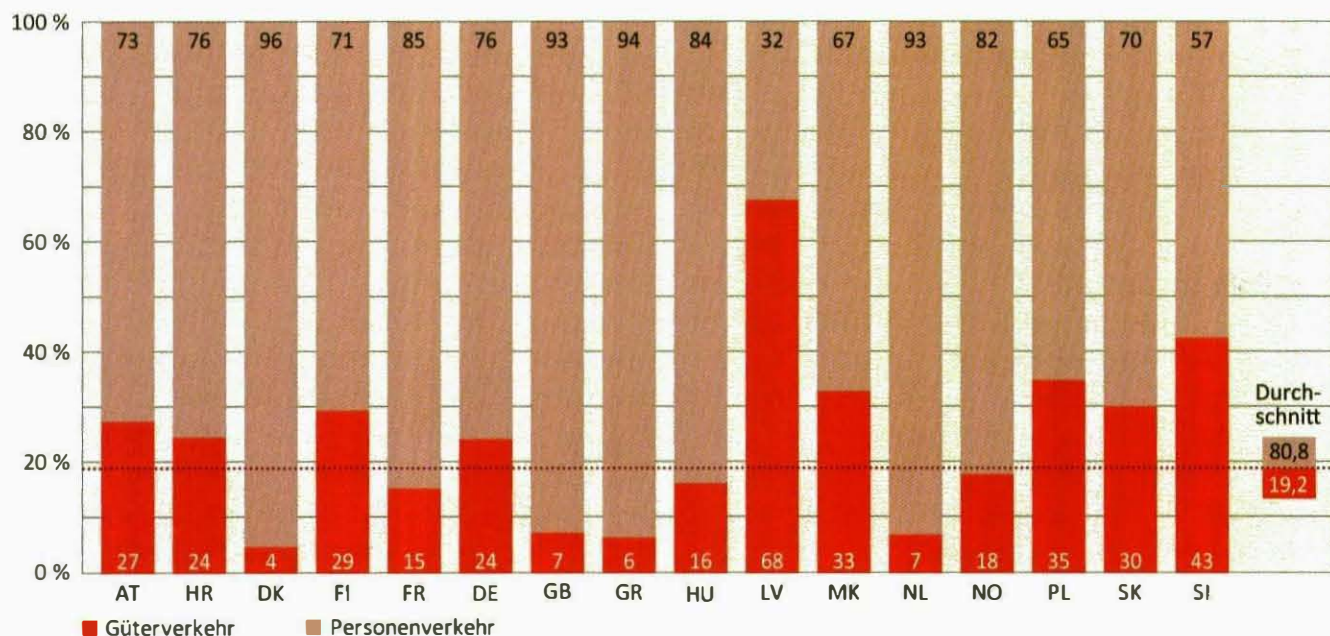
Abb. 2: Nutzung des Schienennetzes. Prozentsätze (Zugkilometer) 2012 für Güterzüge/Personenzüge.
