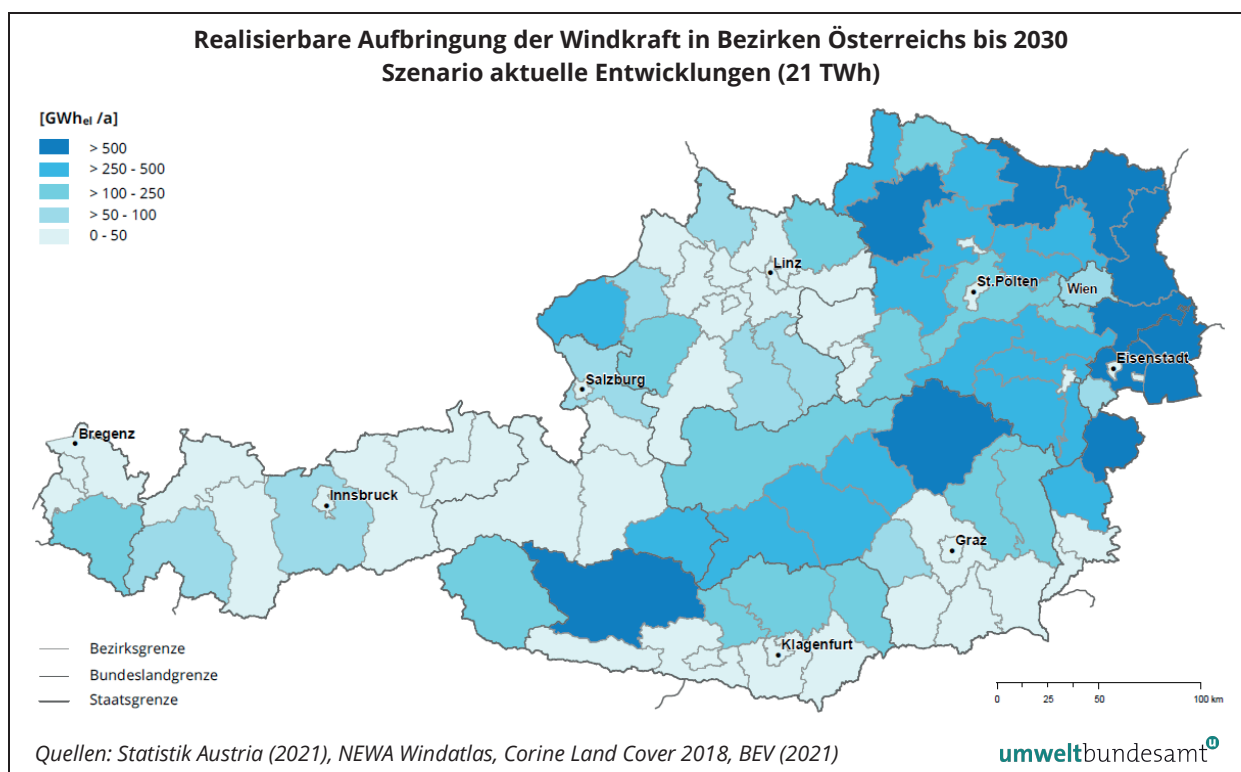
Abbildung 38: Realisierbare Aufbringung der Windkraft in Bezirken Österreichs bis 2030 Szenario aktuelle Entwicklungen (21 TWh), (Umweltbundesamt, 2023b)
