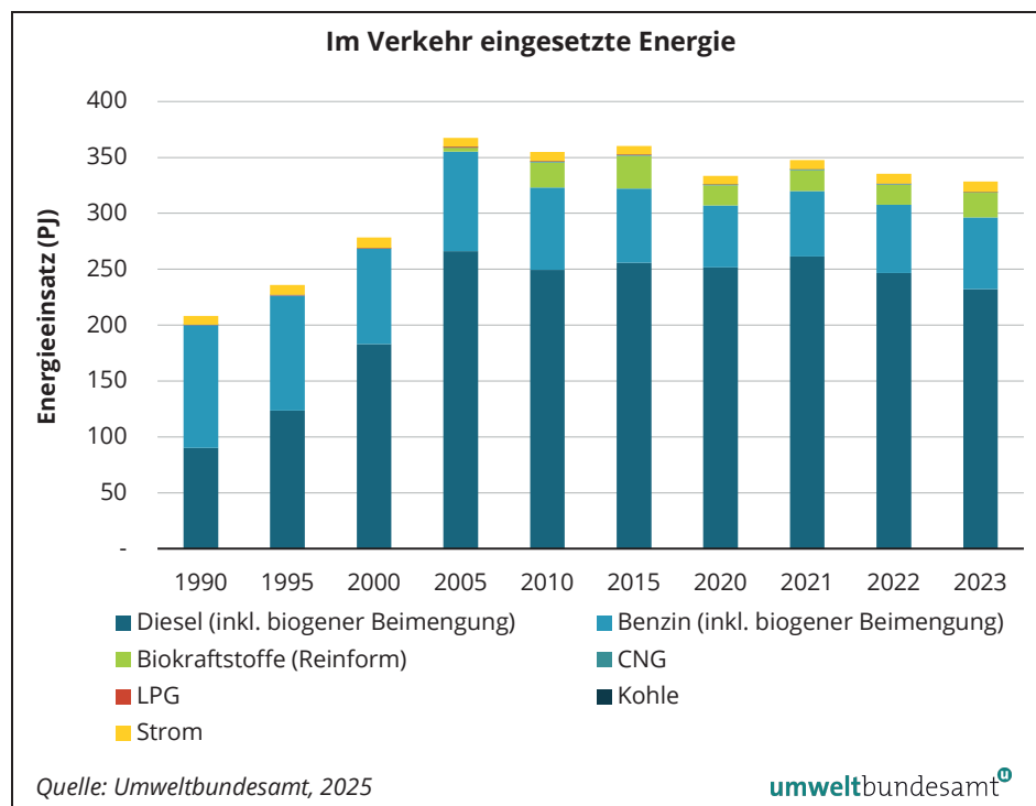
Abbildung 32: Energieeinsatz im Verkehr 1990–2023 in PJ.
