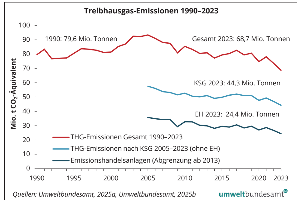
Abbildung 6: Verlauf der österreichischen Treibhausgas-Emissionen 1990–2023.
