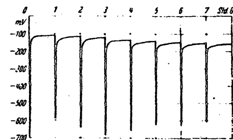
Abb. 2. Ruhepotential des Amalgams, Ag-arm, poliert, in Polyphosphatkalium, gemessen gegen Kalomel, nach jeder Stunde wurde die Deckschicht beseitigt.
