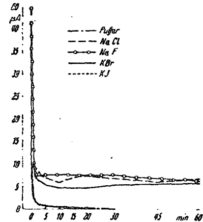
Abb. 4. Stromfluß zwischen Gold- und Amalgamprobe (je 20 mm 2 Oberfläche) in verschiedenen Elektrolyten.
