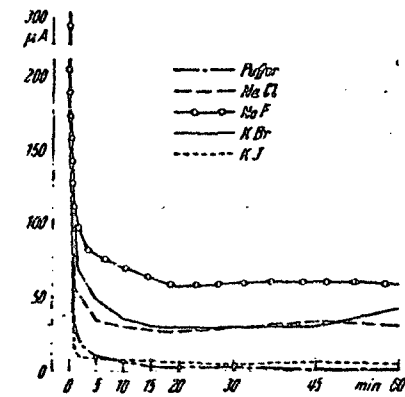
Abb. 4. Stromfluß zwischen Gold- und Amalgamprobe (je 20 mm 2 Oberfläche) in verschiedenen Elektrolyten.
