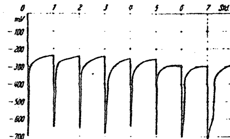
Abb. 1. Ruhepotential des Amalgams, Ag-arm, unpoliert in Polyphosphatkalium, gemessen gegen Kalomel, nach jeder Stunde wurde die Deckschicht beseitigt.
