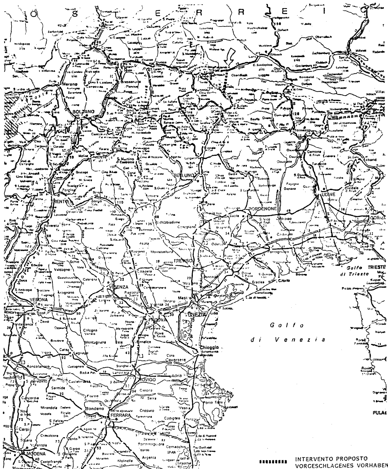
TRAFORO MONTE CAVALLINO RETE STRADALE
