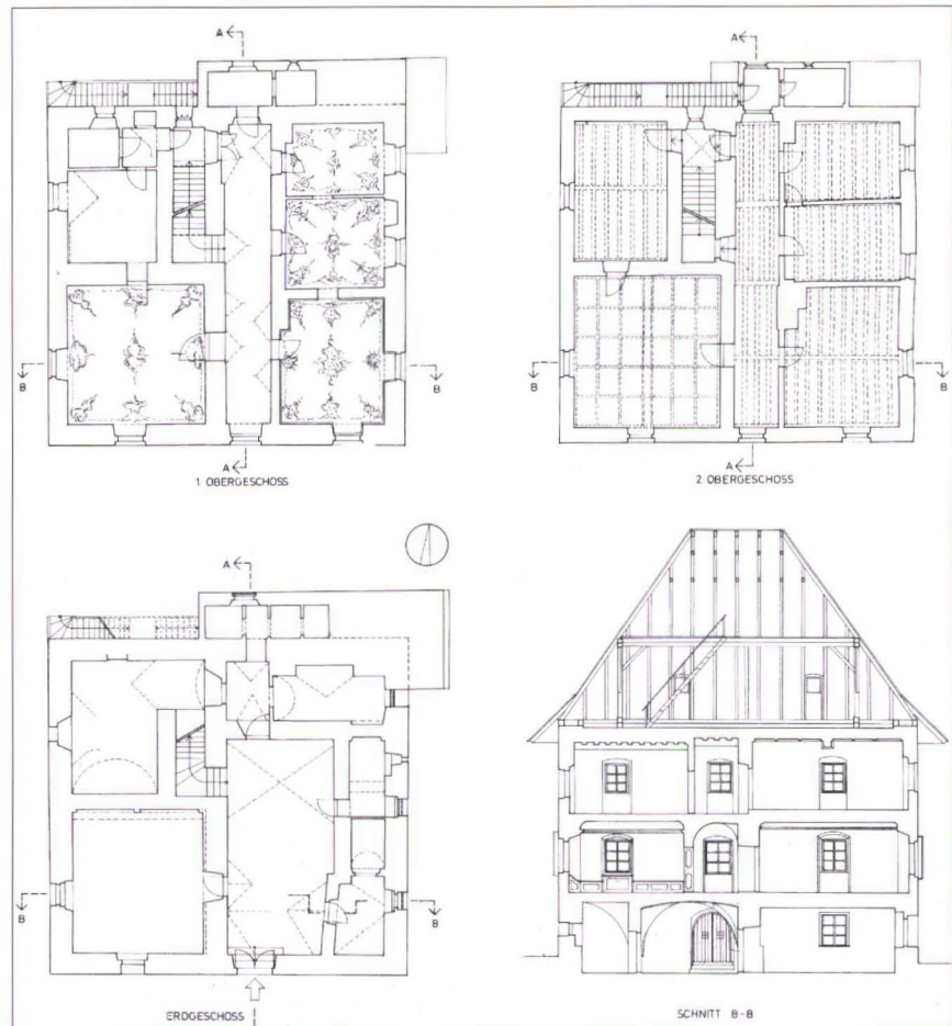
Abb. 1: Lieding, Kärnten, Pfarrhof; Bauaufnahme
