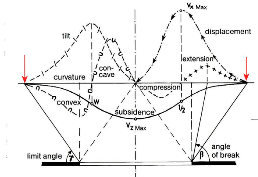
Abb. 30: Darstellung der Senkungsmulden über einem Abbau: die roten Pfeile markieren die Nulllinien. aus: KRATZSCH, H. 1983 (ergänzt)
