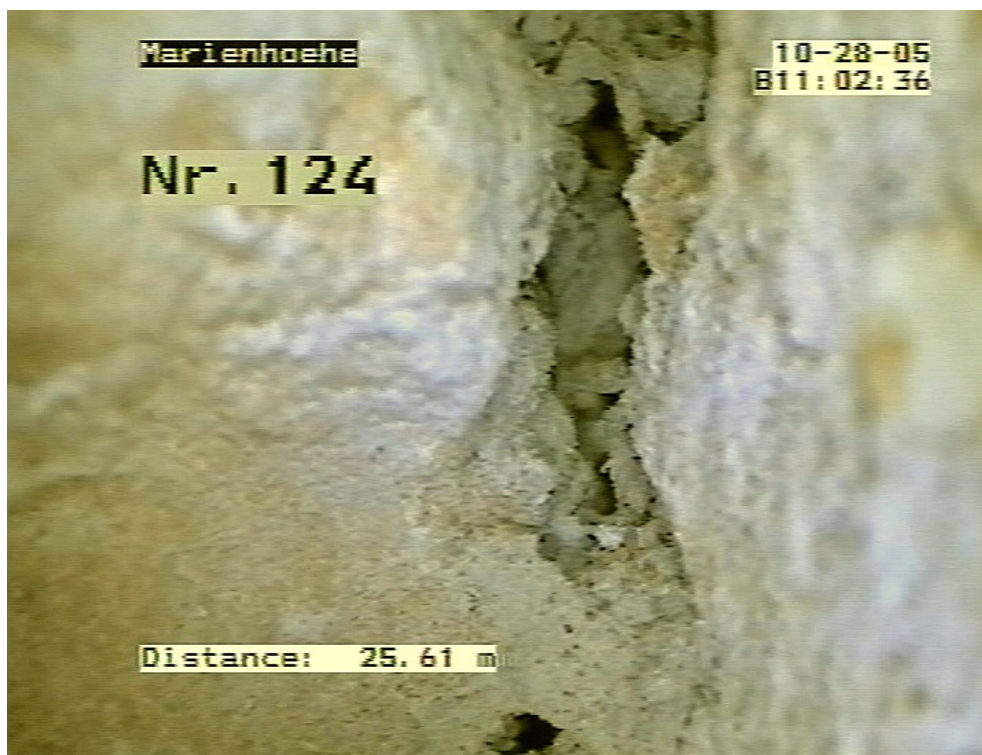
Abb. 9: offene Kluft mit möglichem Betonversatz aus der Sicherungskampagne 2000
