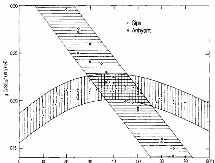
Fig. 2: Abhängigkeit der Löslichkeit von Gips und Anhydrit von der Temperatur (nach H.-J. VOIGT, 1990, aus H. PRINZ 1991).
