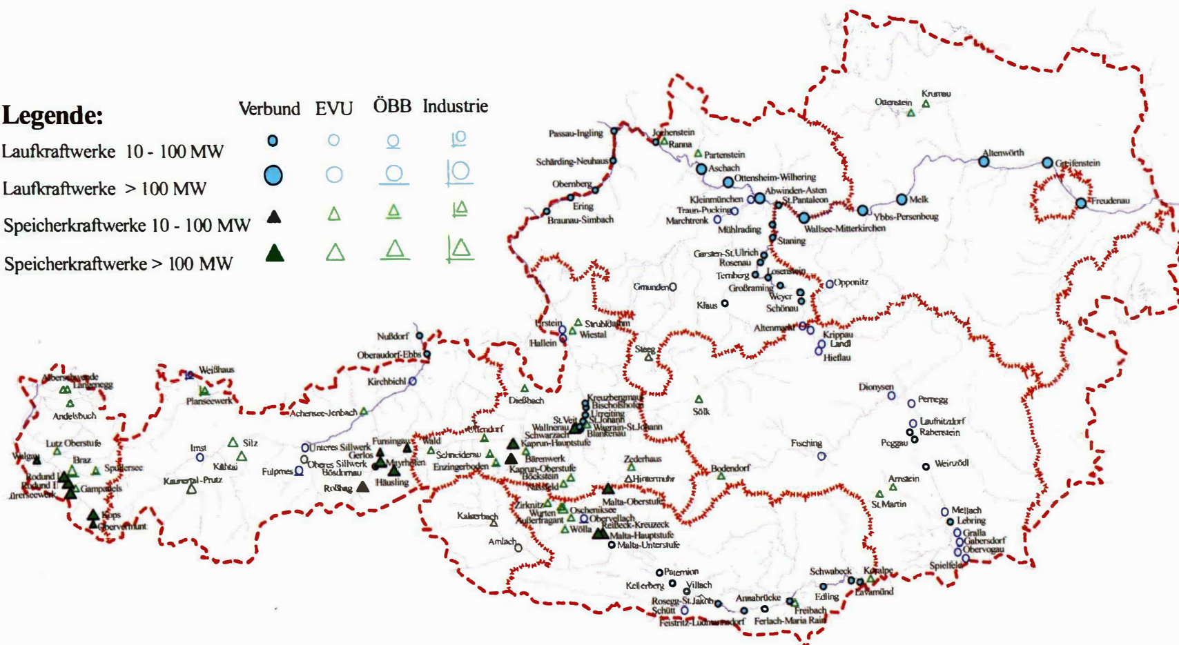
Abbildung 3-13: Wasserkraftwerke > 10 MW in Österreich, Stand 31.12.2001 (Quelle: Verbund)
