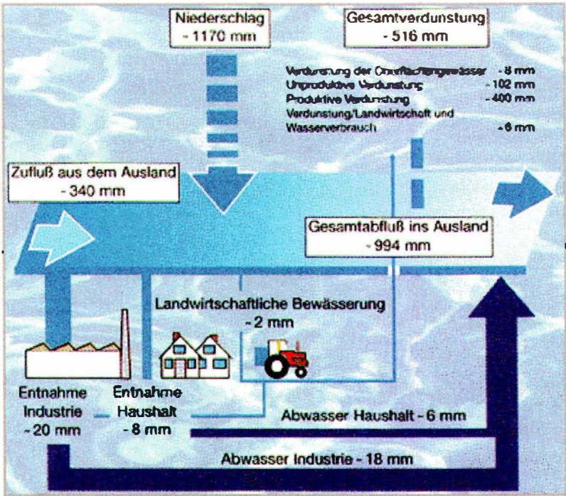
Abbildung 2-4: Wasserbilanz Österreichs
