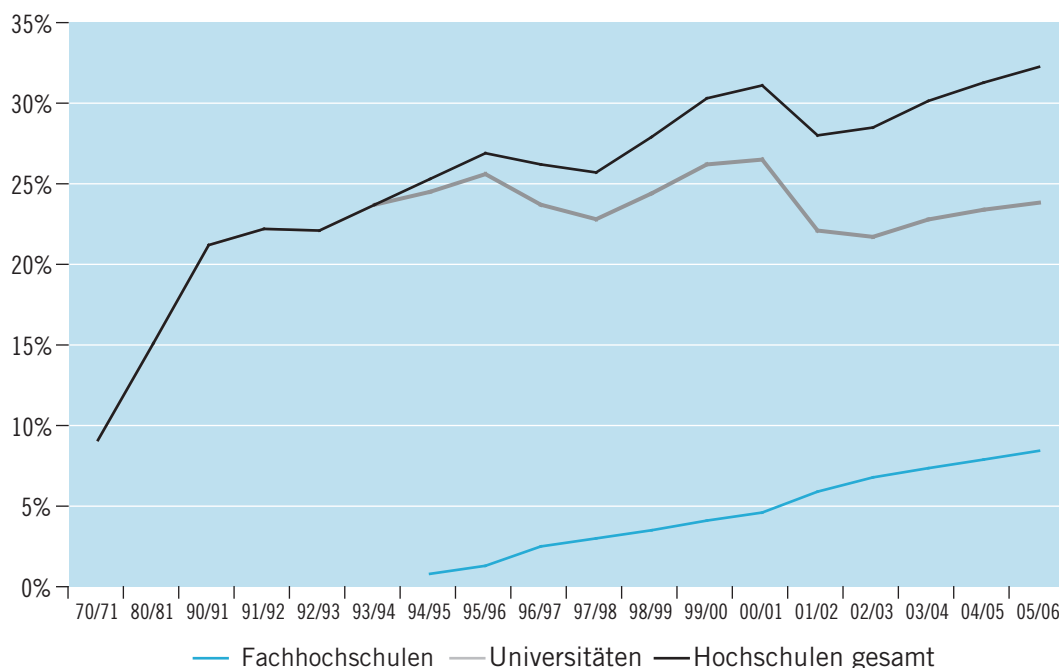
Abbildung 1: Hochschulzugangsquote
