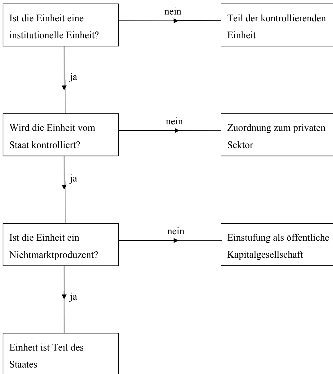
Abbildung 20.1 — Entscheidungsbaum
