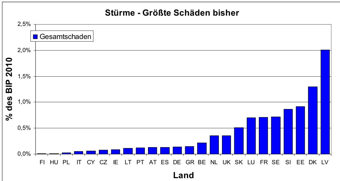
Schaubild 3: Stürme – Größte Schäden bisher
