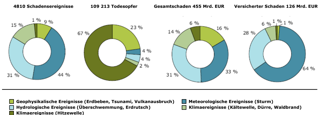
Schaubild 5: Naturkatastrophen in EWR-Staaten — Schadensereignisse, Todesopfer und Verluste (1980 bis 2011)
