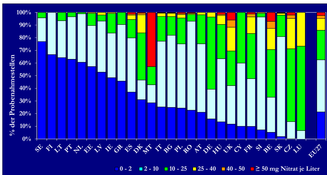
Schaubild B. Häufigkeit der durchschnittlichen Nitratkonzentrationen in Oberflächensüßwasserarten (Jahresdurchschnitt der Nitratkonzentrationen).
