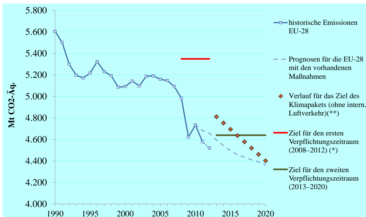
Abbildung 2: Tatsächliche Emissionen (Mt CO 2 -Äquivalent) der EU-28 (ohne internationalen Luftverkehr und LULUCF).
