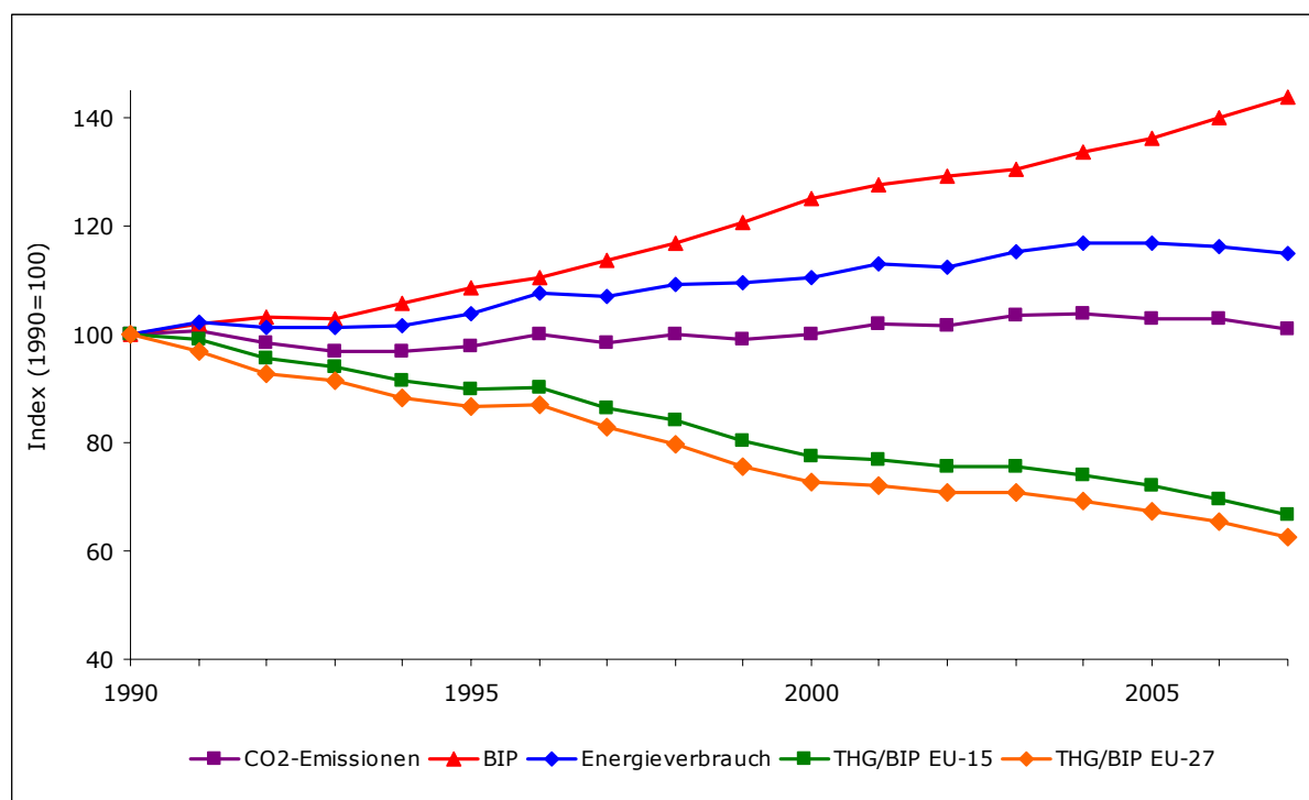
Abbildung 3: Treibhausgasintensitäten für die EU-15 und EU-27, BIP, Energieverbrauch und CO 2 -Emissionen für die EU-15
