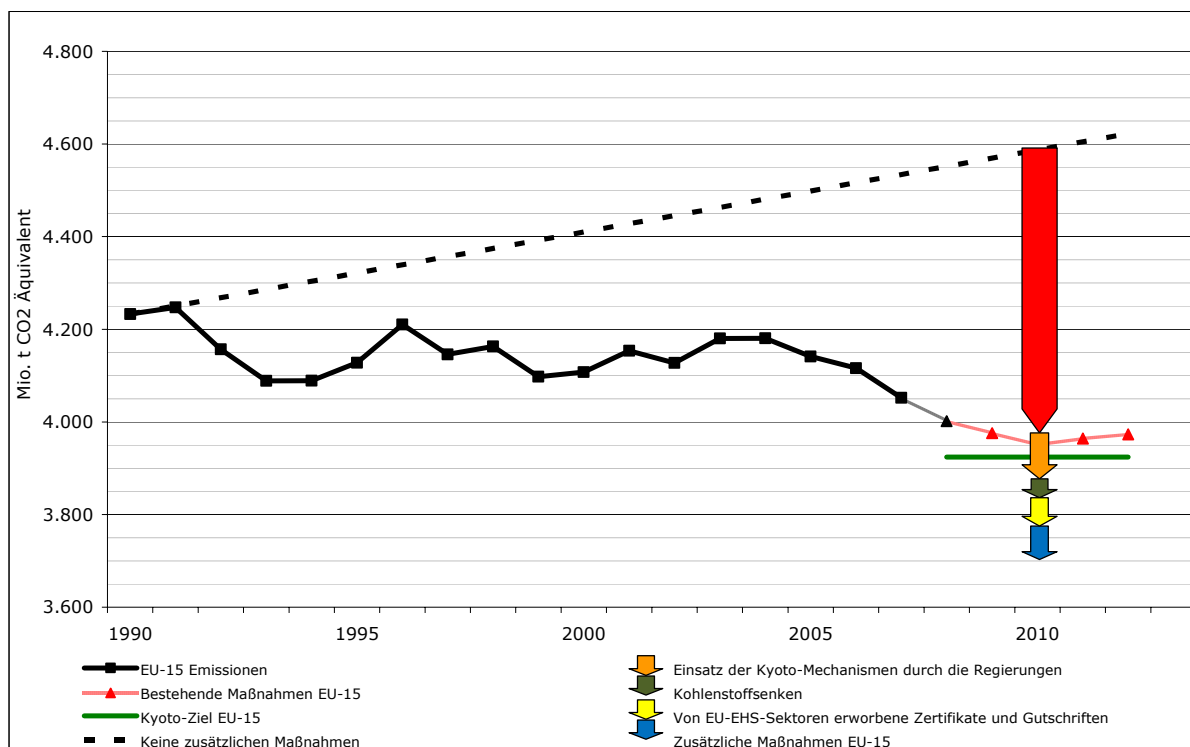
Abbildung 1: Tatsächliche und prognostizierte Emissionen für die EU-15
