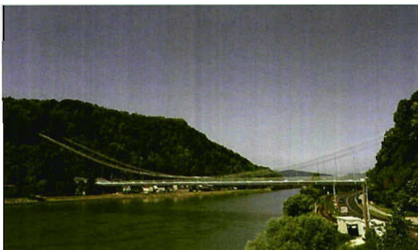
Abbildung 3: Geplante Donaubrücke (Verwirklichungsabschnitt 1)
