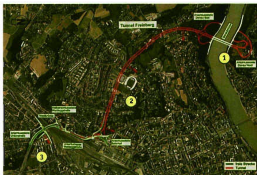
Abbildung 2: Trassenübersicht A 26 Süd, Verwirklichungsabschnitte 1 bis 3 (TZ 20)
