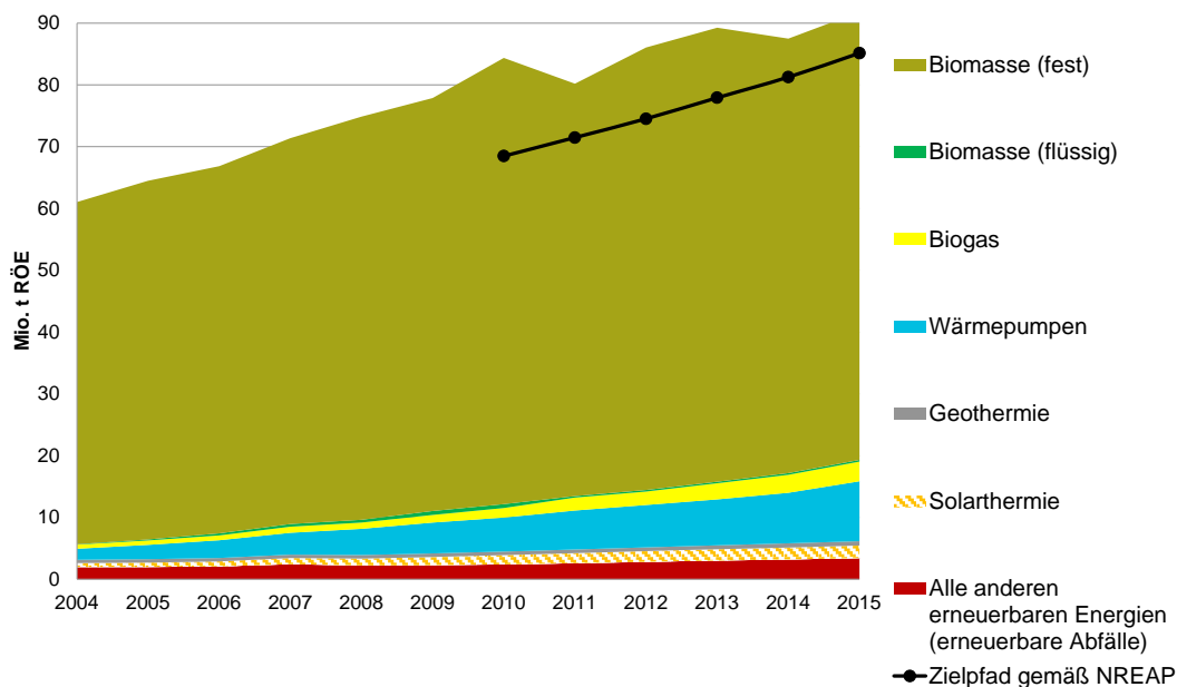
Schaubild 3: Wärme- und Kälteerzeugung in der EU-28 nach Energiequellen (Quelle: EUROSTAT, Öko-Institut)
