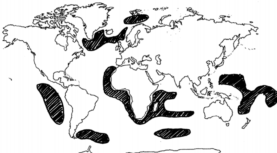
Figure 1: Cartographie sommaire de la répartition potentielle des activités de pêche de la flotte de pêche externe de l'Union européenne.
