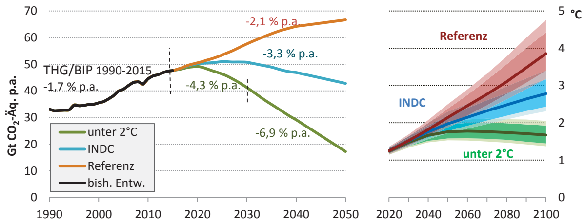
Abbildung 11: Weltweite Emissionen (Gt CO 2 -Äq.) und prozentuale Veränderung der Emissionsintensität pro BIP-Einheit (links). Globaler durchschnittlicher Temperaturanstieg (rechts). 42
