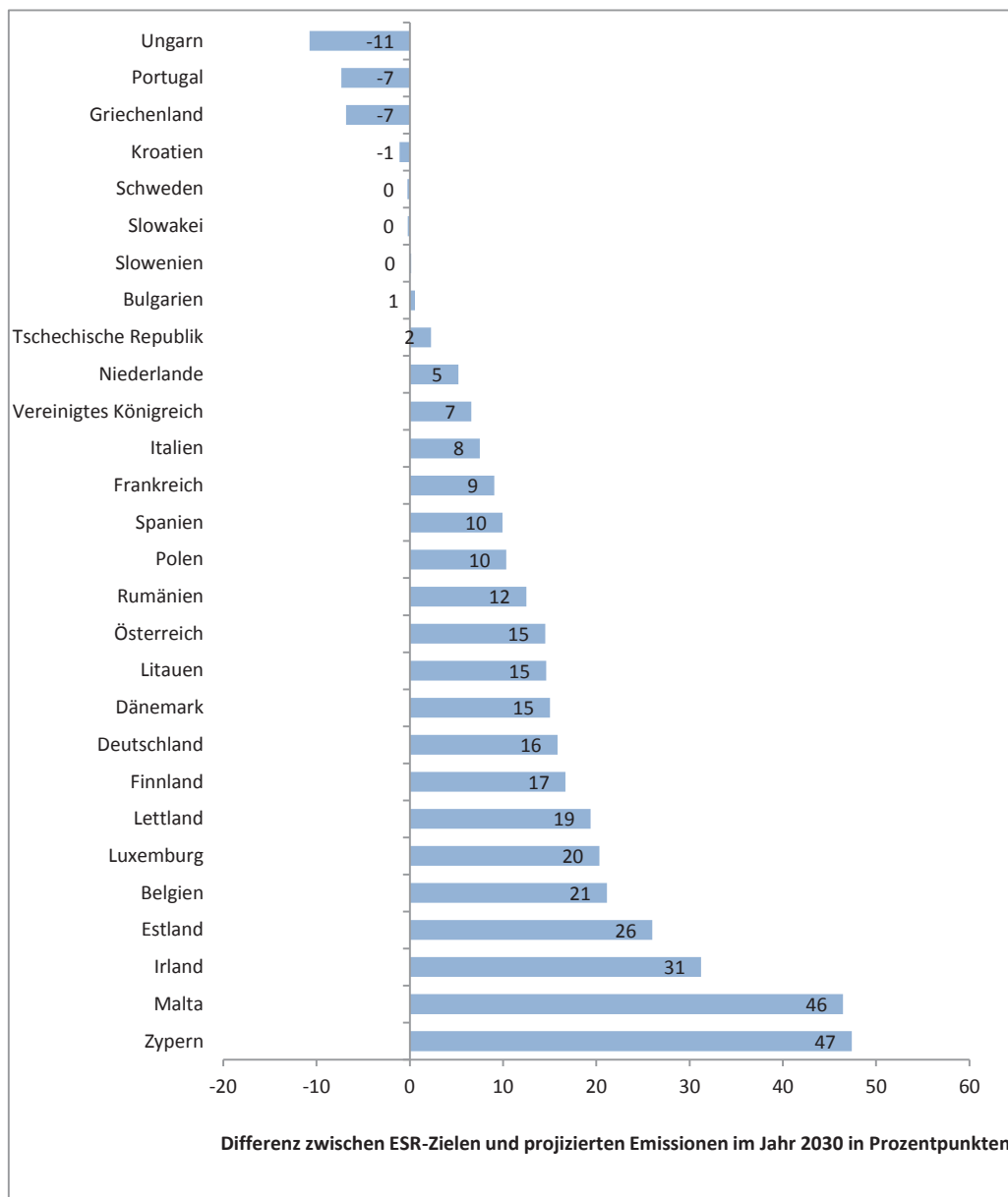
Abbildung 6: Differenz zwischen den Zielen der Lastenteilungsverordnung bis 2030 und den projizierten Emissionen (Prozentpunkte). 15 (Negative Werte weisen darauf hin, dass
