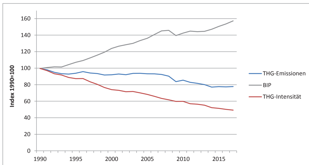
Abbildung2: THG-Emissionen in der EU, reales BIP und THG-Emissionsintensität (1990 = 100). 2
