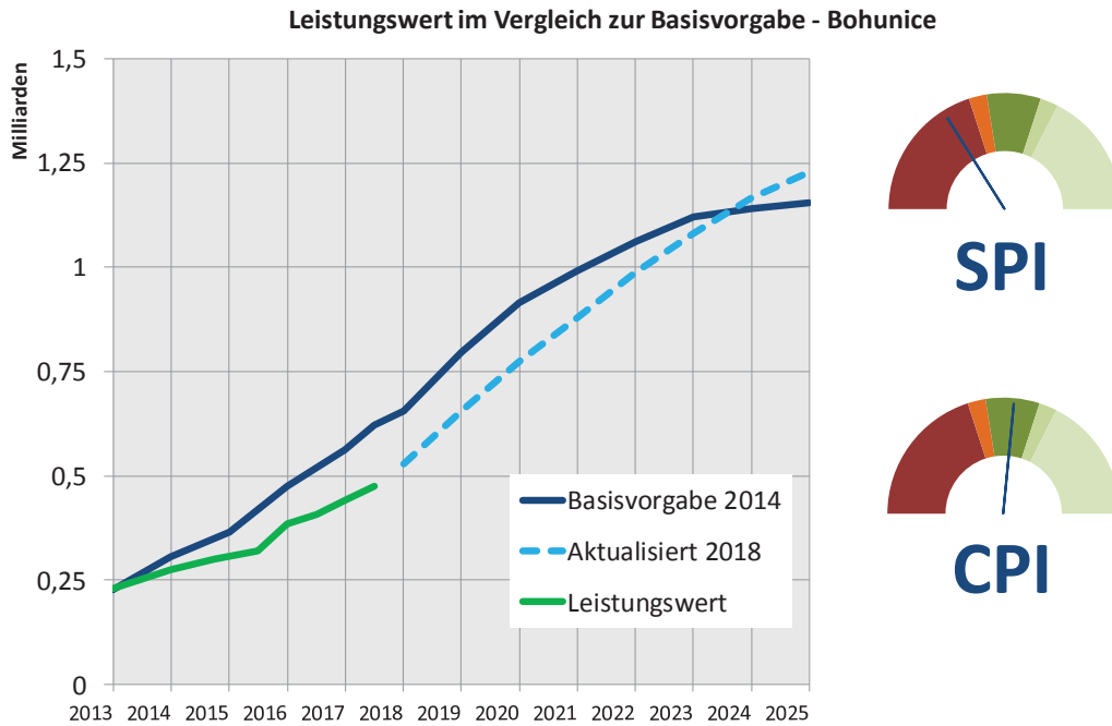
Abbildung 4 Anhand des „Leistungswert-Management“-Systems gemessener Fortschritt und gemessene Leistung. Die dargestellten Werte umfassen keine Rückstellungen für unvorhergesehene Ausgaben. Die Gesamtkostenschätzung (einschließlich Rückstellungen für unvorhergesehene Ausgaben) beläuft sich 2018 auf 1238 Mio. EUR, während sie sich 2014 auf 1246 Mio. EUR belief.
