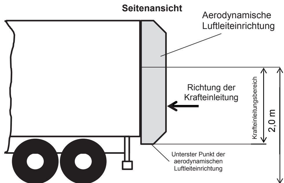
Abbildung 3 Krafteinleitung
