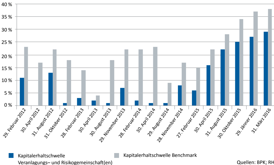
Abbildung 6: Unterschreitungswahrscheinlichkeit der Kapitalerhaltsschwelle
