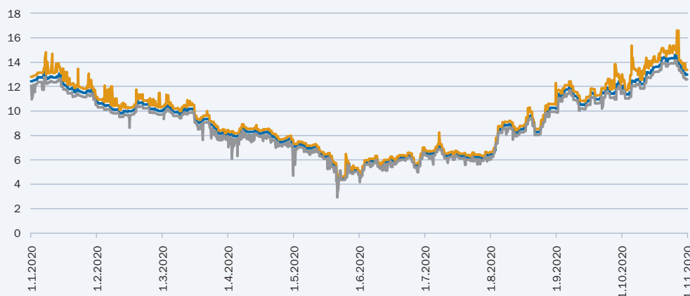
PREISE FÜR STUNDENBILANZIERENDE BILANZGRUPPEN – MG OST in EUR/MWh
