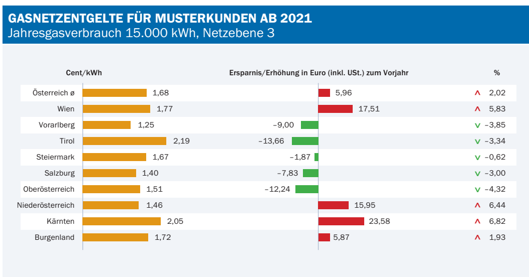
Abbildung 23 Gasnetzentgelte (Netzebene 3) für Musterkunden 2021 mit Vergleich zu 2020
