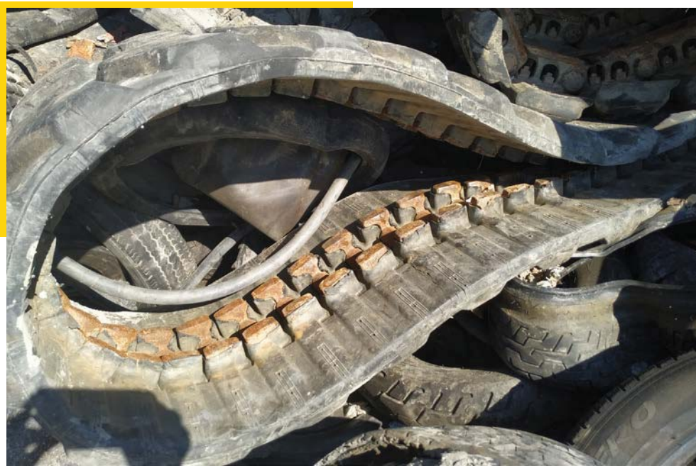
Abbildung 143: Baggerketten-Gummiabfälle mit sehr hohem Metallgehalt, schadstoffhaltig – nicht gelisteter Abfall
