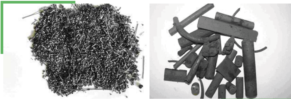
Abbildung 265: Wolframhaltiger-Pressbruch
