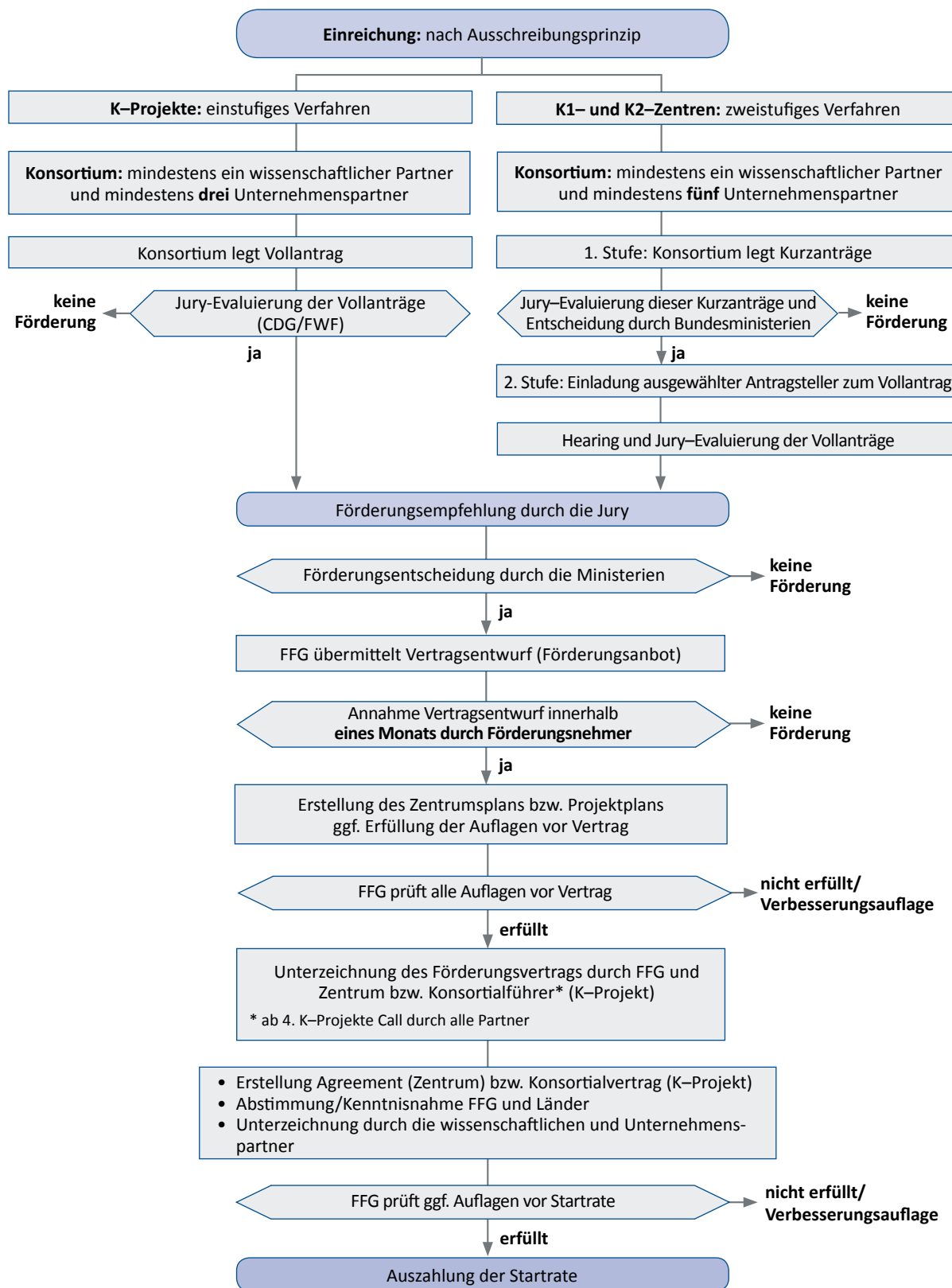
Abbildung 4: Programmablauf
