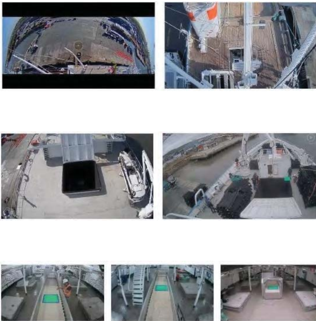
Abbildung 1: (A) Beispiel für ein auf einem Ringwadenfänger installiertes EM-System mit 6 Kameras, das die wichtigsten Bereiche für Fischfang und Fischhandhabung erfasst (entnommen aus Murua et al., 2020b) und (B) auf einem Ringwadenfänger installiertes EM-System mit 7 Kameras (4 auf dem oberen Deck und 3 auf dem Welldeck), das die wichtigsten Bereiche für Fischfang und Fischhandhabung erfasst, einschließlich einer weiteren Kamera am Förderband: (B1) 360°-Panoramakamera (z. B. Sicht auf Backbord), (B2) Kamera im Ausguck mit Hecksicht, (B3) Sicht auf den Deckkran auf dem Arbeitsdeck, (B4) Vordeck-Bildkamera, (B5) Sichtfeld der Förderband-Heckkamera, (B6) Förderband-Mittelkamera und (B7) Förderband-Bugkamera (Quelle: Digital Observer Services).
