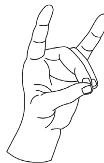
Abb. 4.8.: „Wolfszeichen“/„Wolfsgruß“
